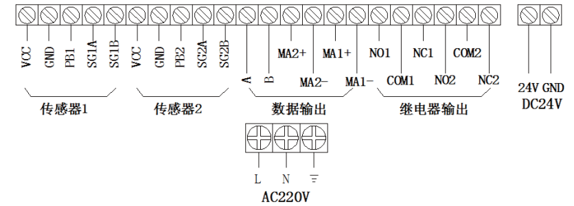
变送器接线端子图
