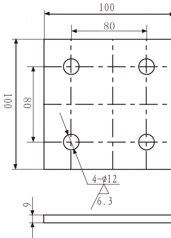
附录一：固定底座尺寸图
