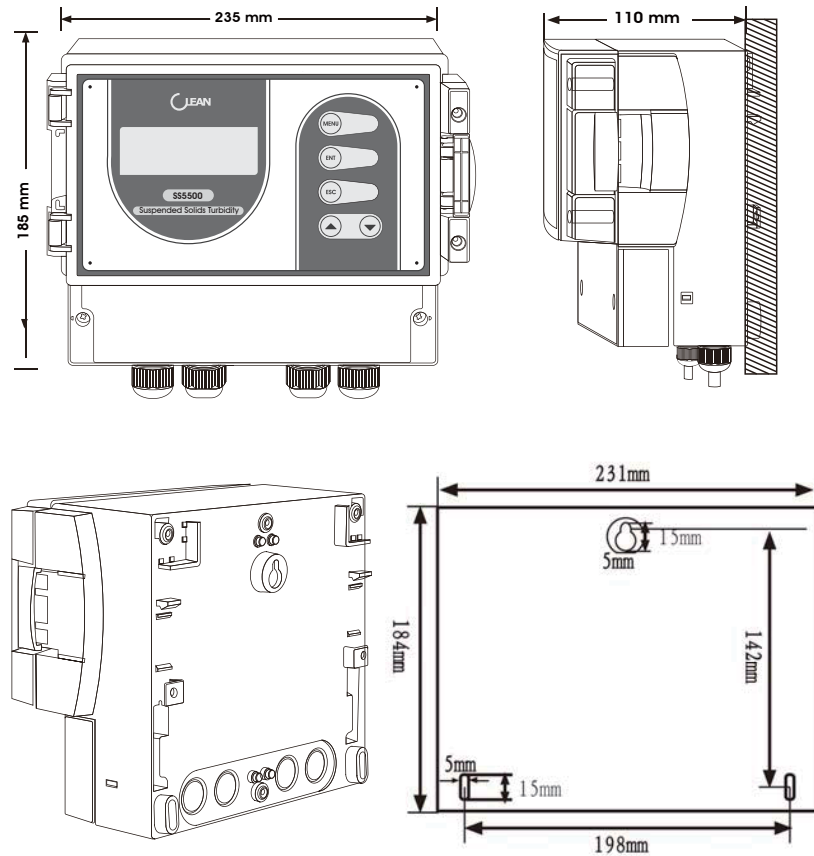
外形尺寸
